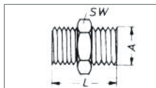
Racor Cupla macho
