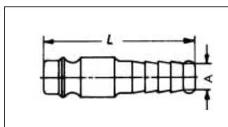
Racor manguera
