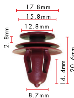
Grapa TPC Modelo: GM 30006620 TOYOTA 67771-12050, 67771-28020 Art. No. 0500920221
