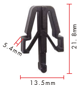
Grapa negra de rejilla Para tapón de la alameda Modelo: TOYOTA / MAZDA / G.M ISUZU / 22mm x 13mm Art. No. 0500920071
