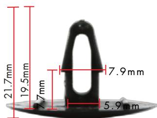
Remache impato negro Se adapta a un agujero de 8mm Modelo: TOYOTA Art. No. 0500920092
