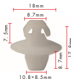
Grapa doble Modelo: TOYOTA 90467-11063 PREVIA 1990-ON Art. No. 0500920106
