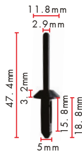
Remache plástico Modelo: GM 20423647 FORD N804189S Art. No. 050113754
