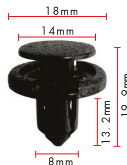
Grapa mini negra de presión de punta cónica Modelo: NISSAN 01553-09611, 01553-10501, 90467-08185 Art. No. 0500920321
