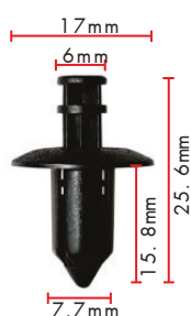
Remache impacto negro Modelo: HONDA / TOYOTA / SUZUKI SUBARU / MITSUBISHI / NISSAN Art. No. 0500920285
