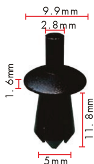
Retenedor de tubo de ventilación inferior Art. No. 0500920029
