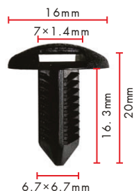
Grapa maletero Modelo: TOYOTA 90467-08186 Art. No. 0500920265
