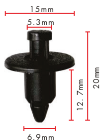
Retenedor tipo empuje Modelo: G.M 96057846 / TOYOTA 90467-07041 / SUZUKI 09409-07308-5PK HYUNDAI / 13mm x 6.3mm Art. No. 0500920057
