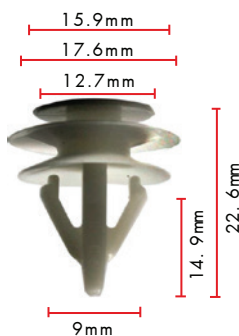
Grapa natural con ganchos para puerta Modelo: HONDA 91566-SPO-003 Art. No. 0500920261
